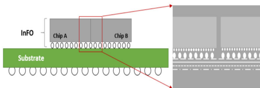
圖三、台灣半導體晶圓代工廠發展之 Info-on-Substrate(InFO-oS)
